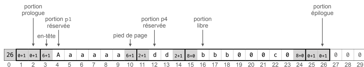
FIGURE 5 – Exemple de contenu de la mémoire après nouvelle réservation - Partie III.
